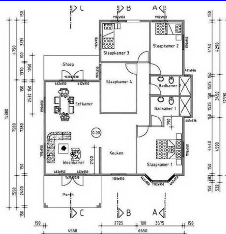
de bouwtekening
